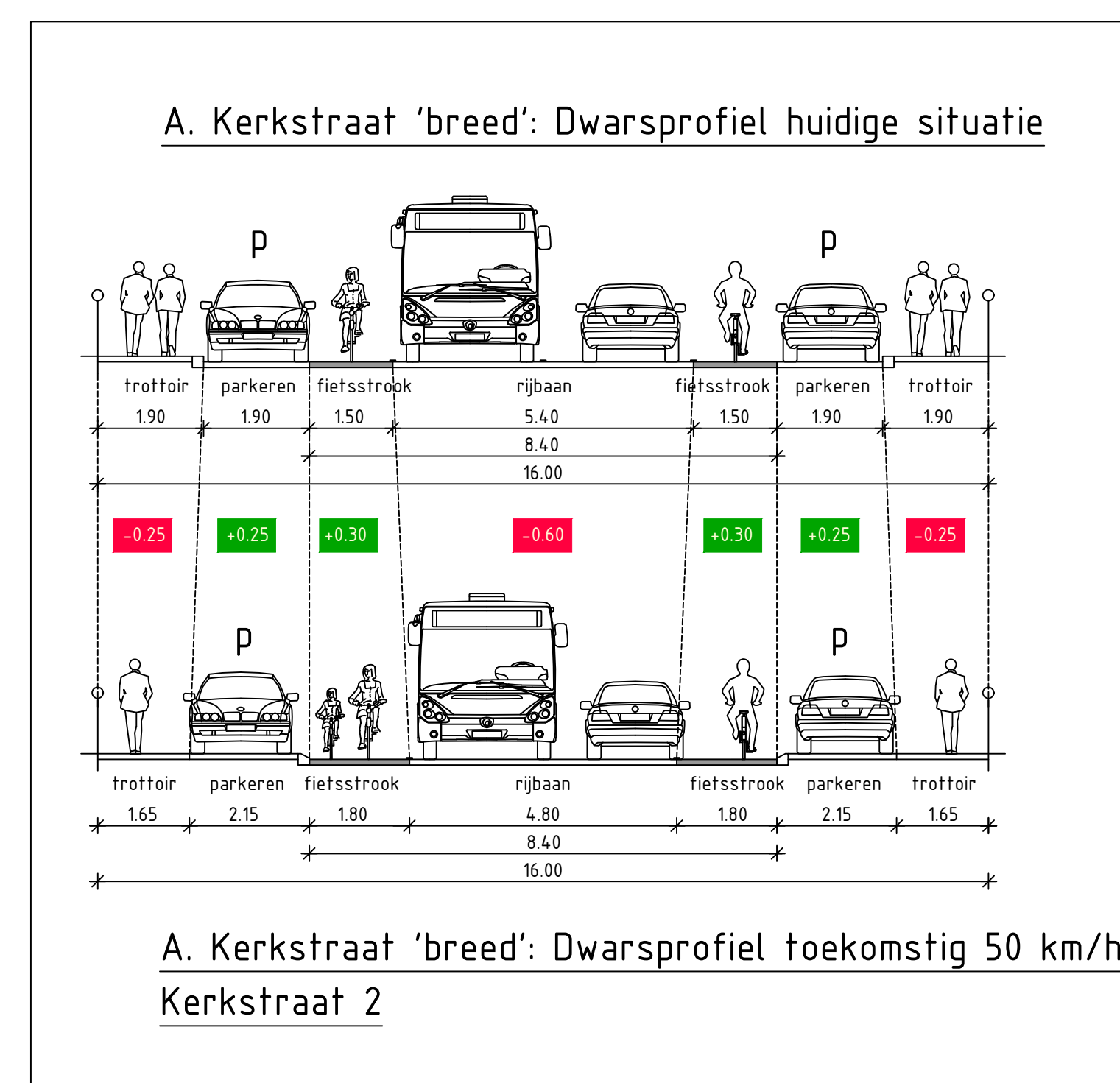
Profiel A
