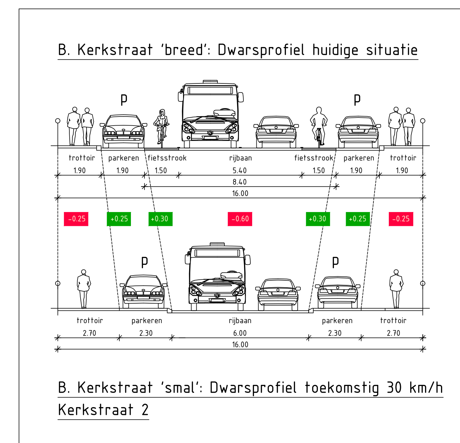
Profiel B
