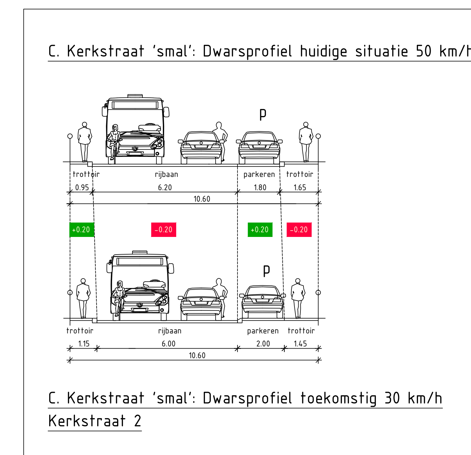
Profiel C
